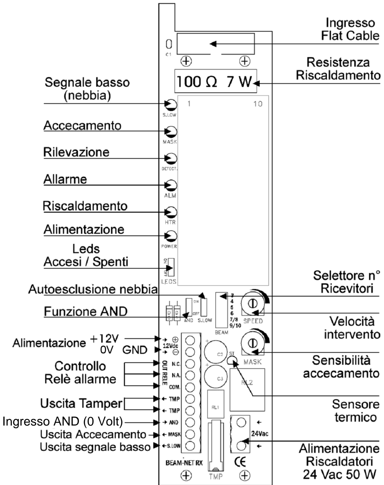
Scheda ricevitori ( RX ) - fig. 1
