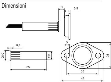
Dimensioni
