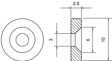
Dimensioni
