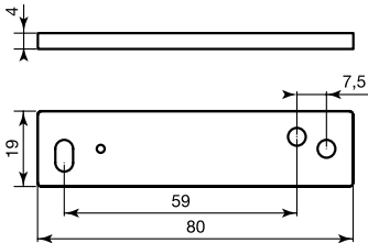
Dimensioni
