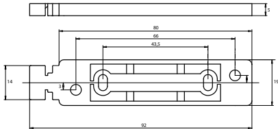
Dimensioni
