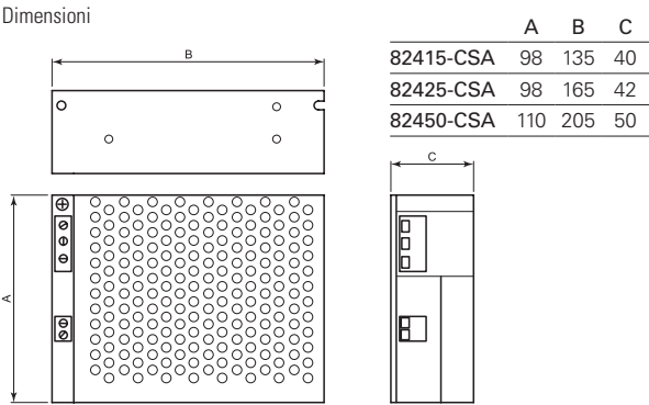
Dimensioni
