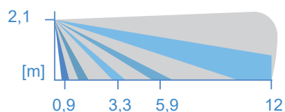
Vista laterale
