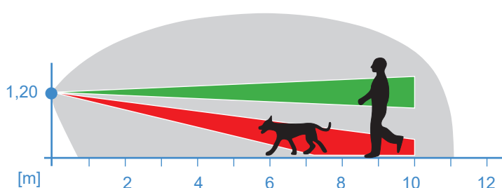
Vista laterale
