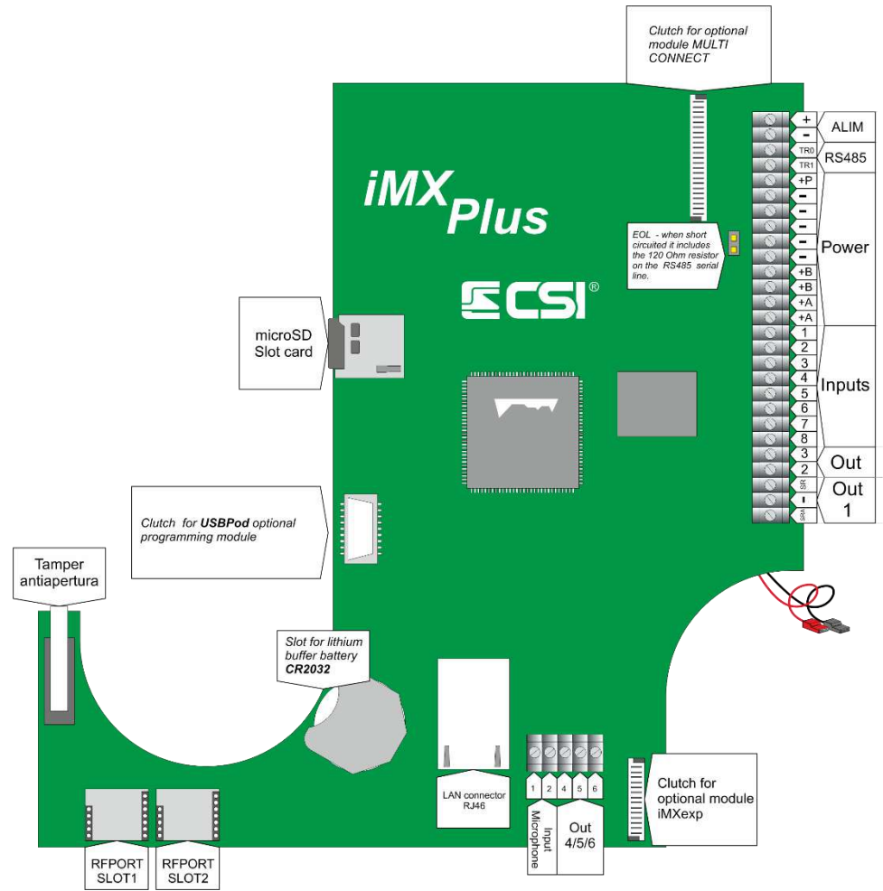
iMX Plus
