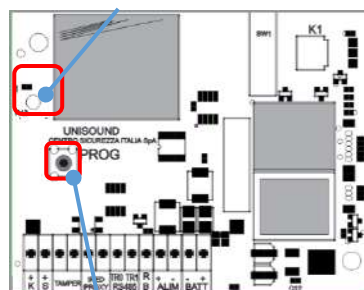
Tasto PROG
