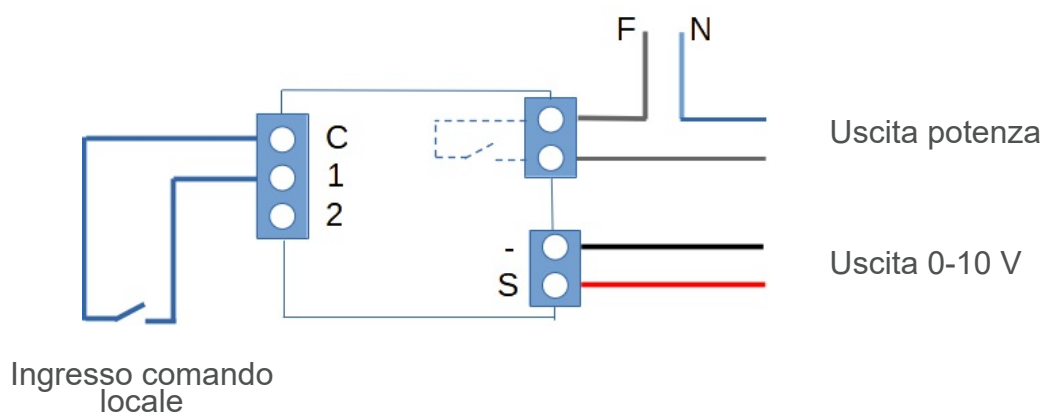
Schema collegamenti utilizzatori
