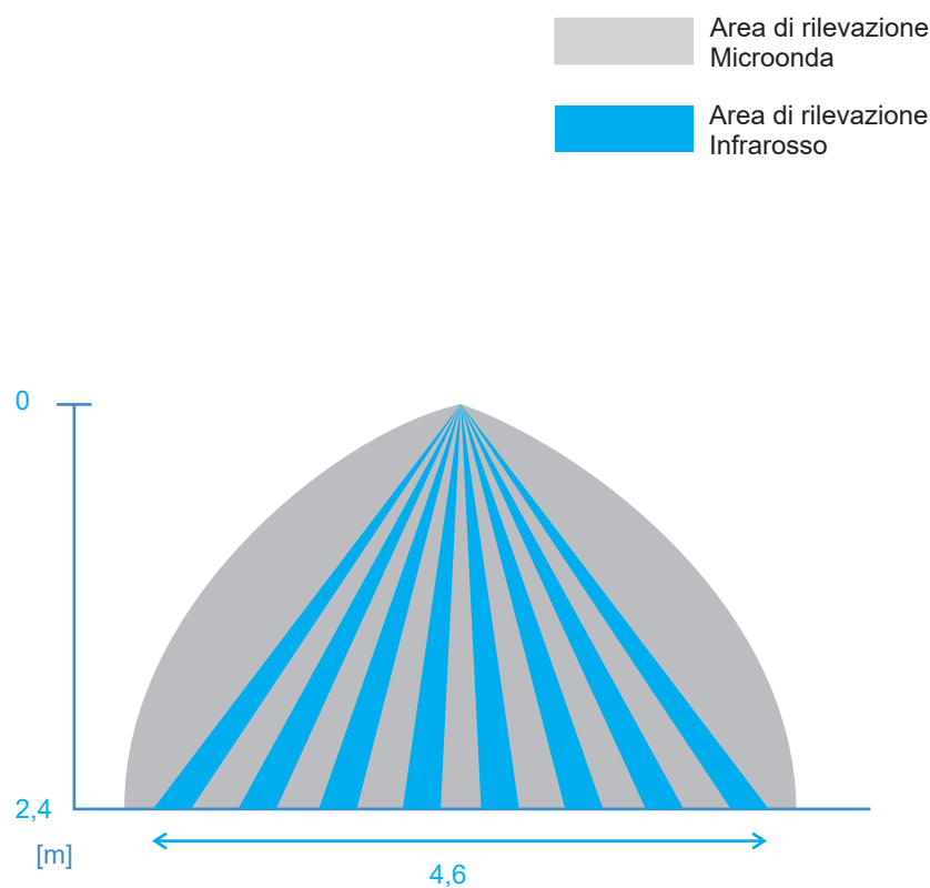
Vista dall'alto
