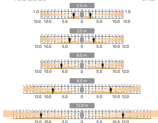
Vista laterale
