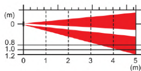
Distanza di rilevazione m5
