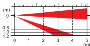
Distanza di rilevazione m2
