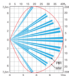
Vista dall'alto
